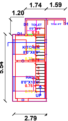
PLAN1
