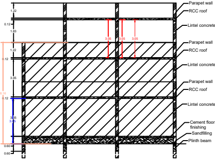
SECTION - AB
