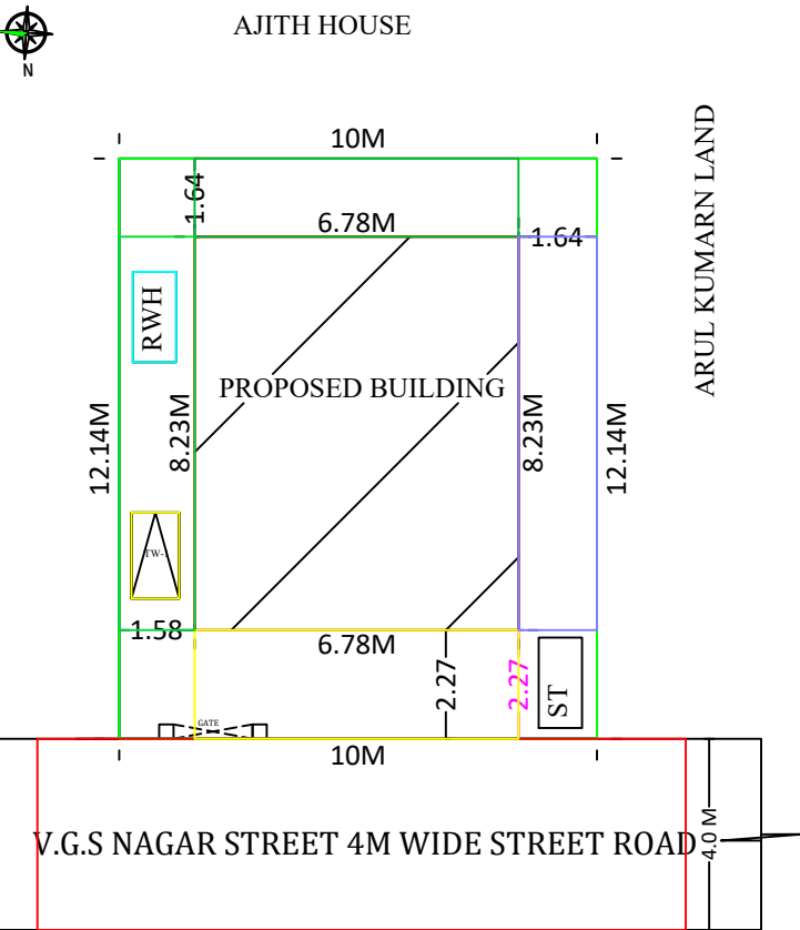
SITE PLAN 1:100 SCALE
