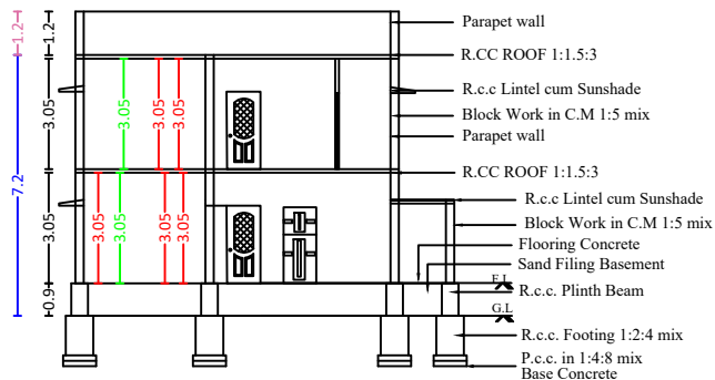
SECTION A-B
