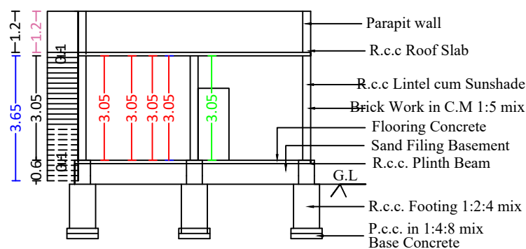
SECTION A-B
