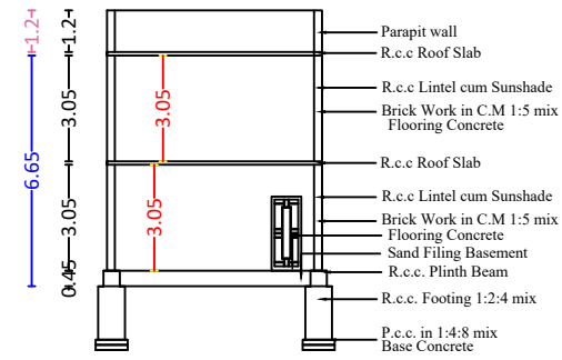
SECTION A-B
