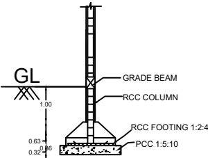
SECTION ON - BB (N.T.S)
