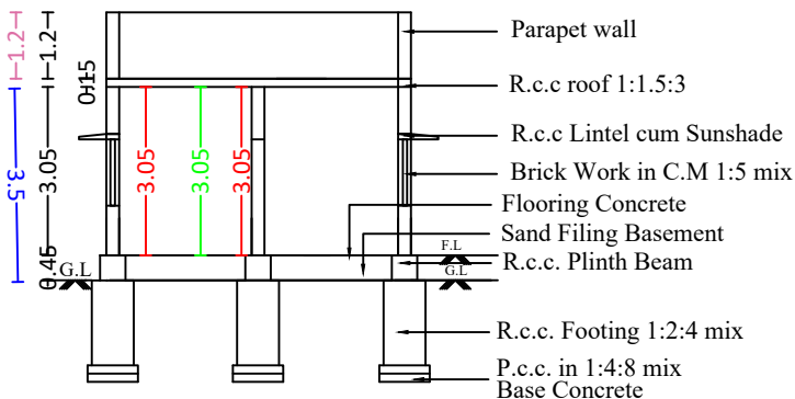
SECTION A-B
