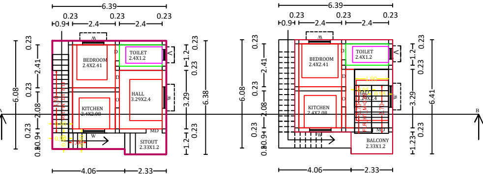
F.F PLAN
