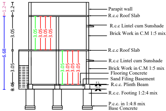
SECTION A-B
