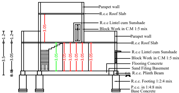
SECTION A-B
