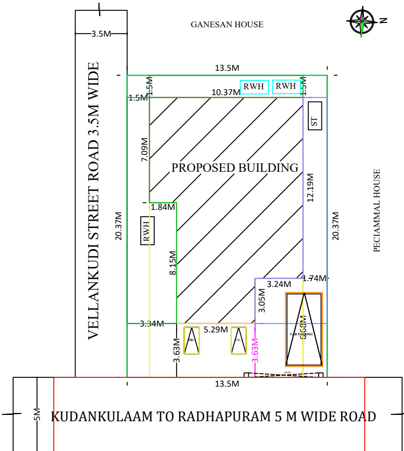
SITE PLAN 1:100 SCALE
