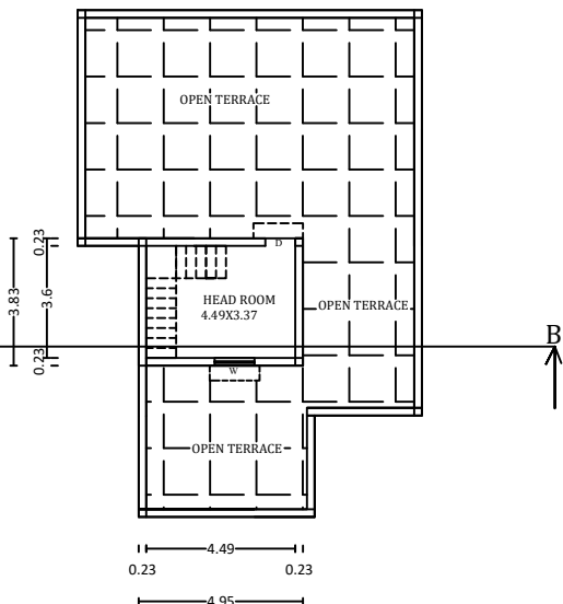
F.F. PLAN
