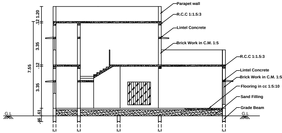
SECTION 'AB'
