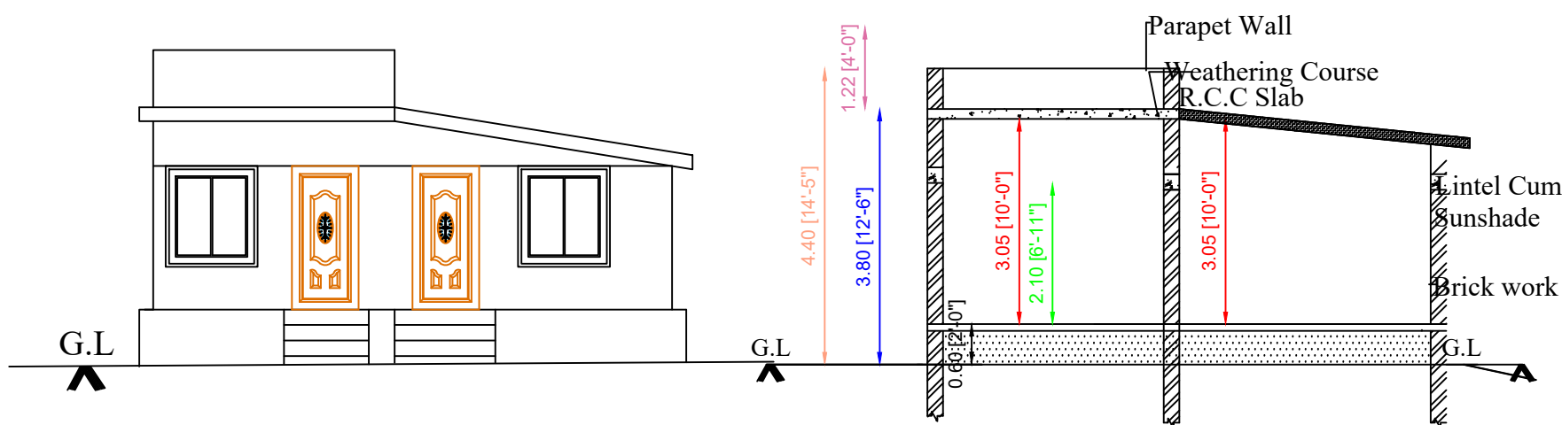
ELEVATION
