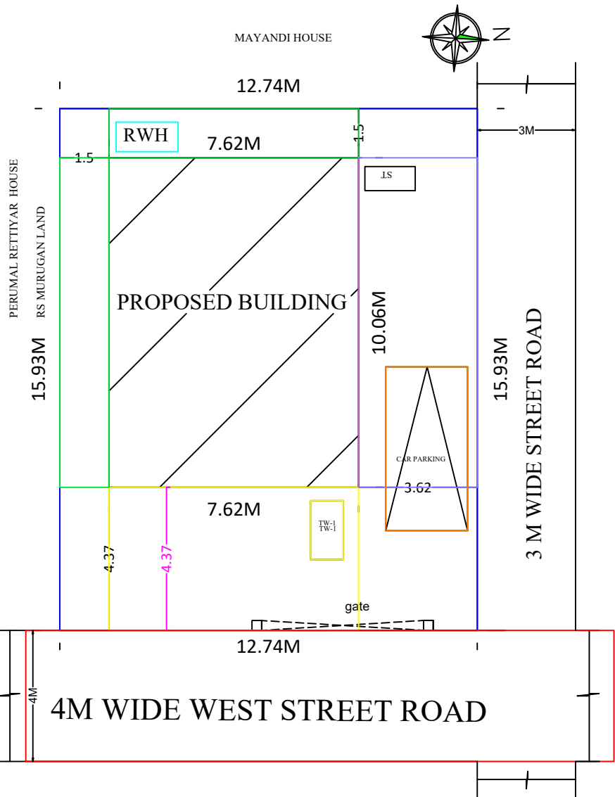
SITE PLAN 1:100 SCALE
