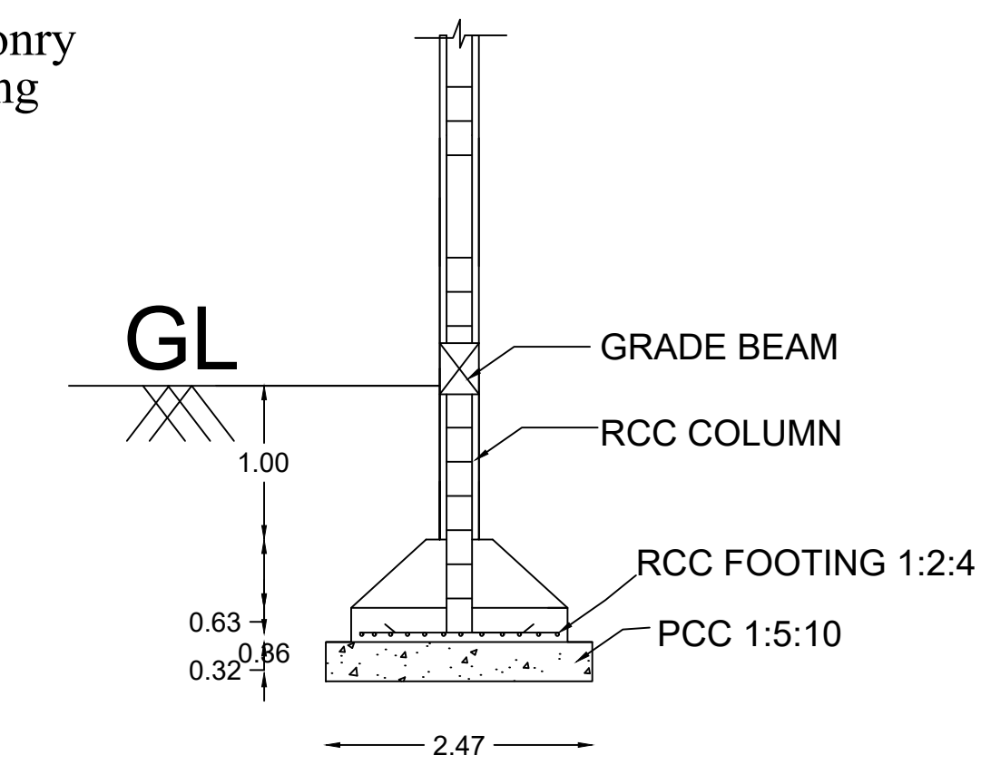
SECTION ON - BB (N.T.S)
