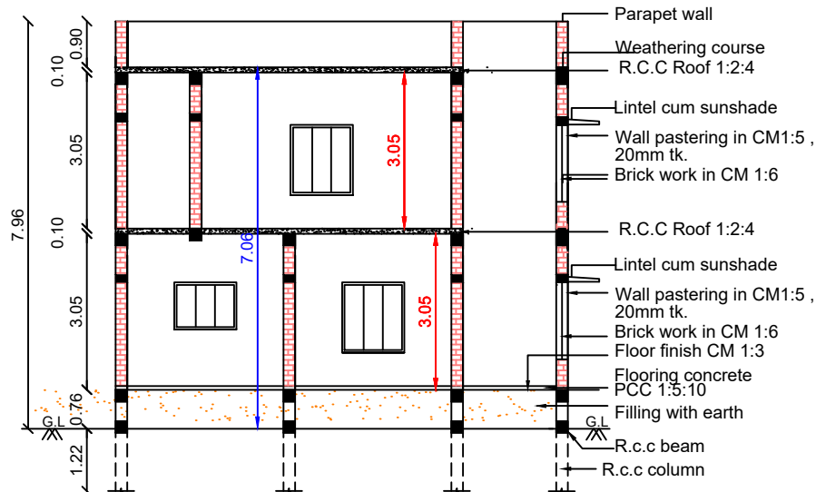
SECTION A-B
