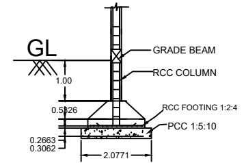
SECTION ON - BB (N.T.S.)
