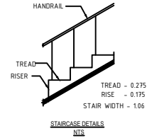
STAIRCASE DETAILS N.T.S
