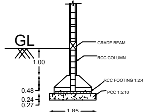
SECTION ON - BB (N.T.S)
