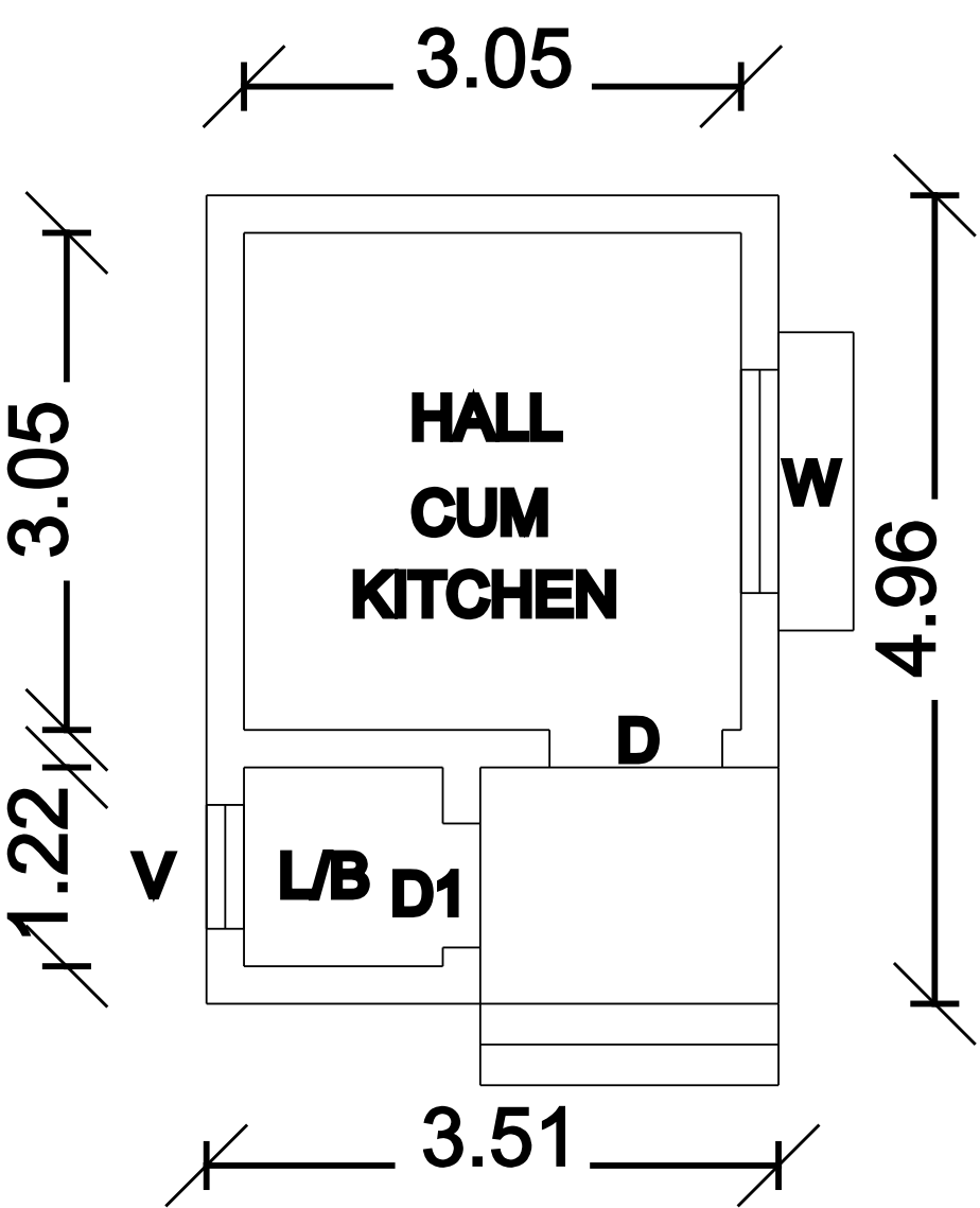
G.F PLAN
