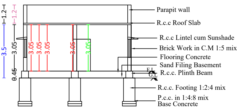
SECTION A-B
