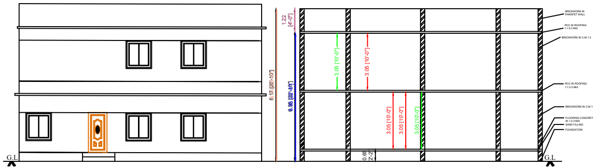
ELEVATION
