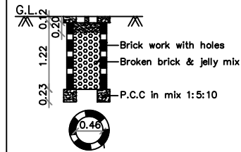
(Scale: - 1:50)
