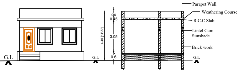
ELEVATION
