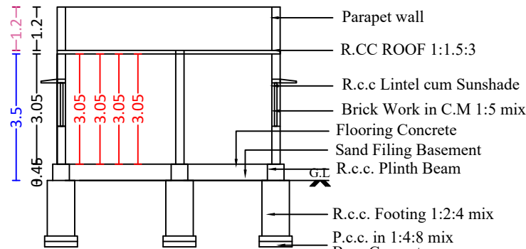
SECTION A-B
