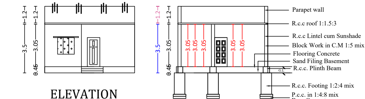
SECTION A-B
