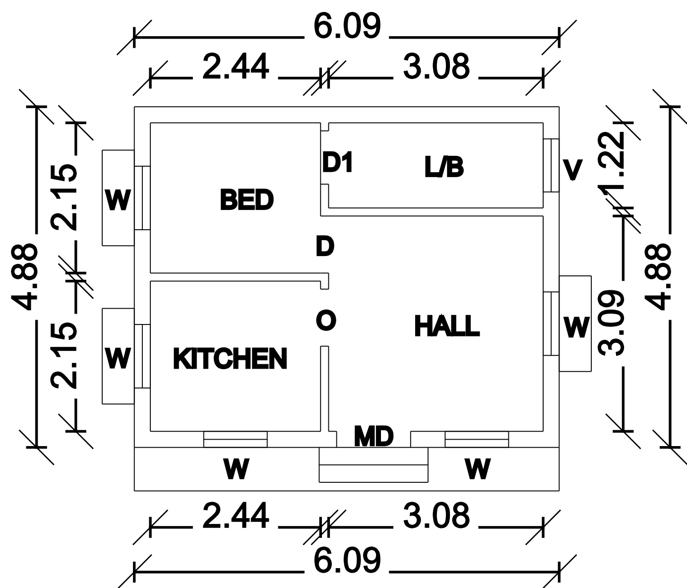
G.F PLAN
