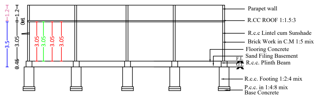
SECTION A-B
