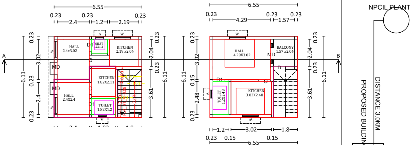
F.F PLAN
