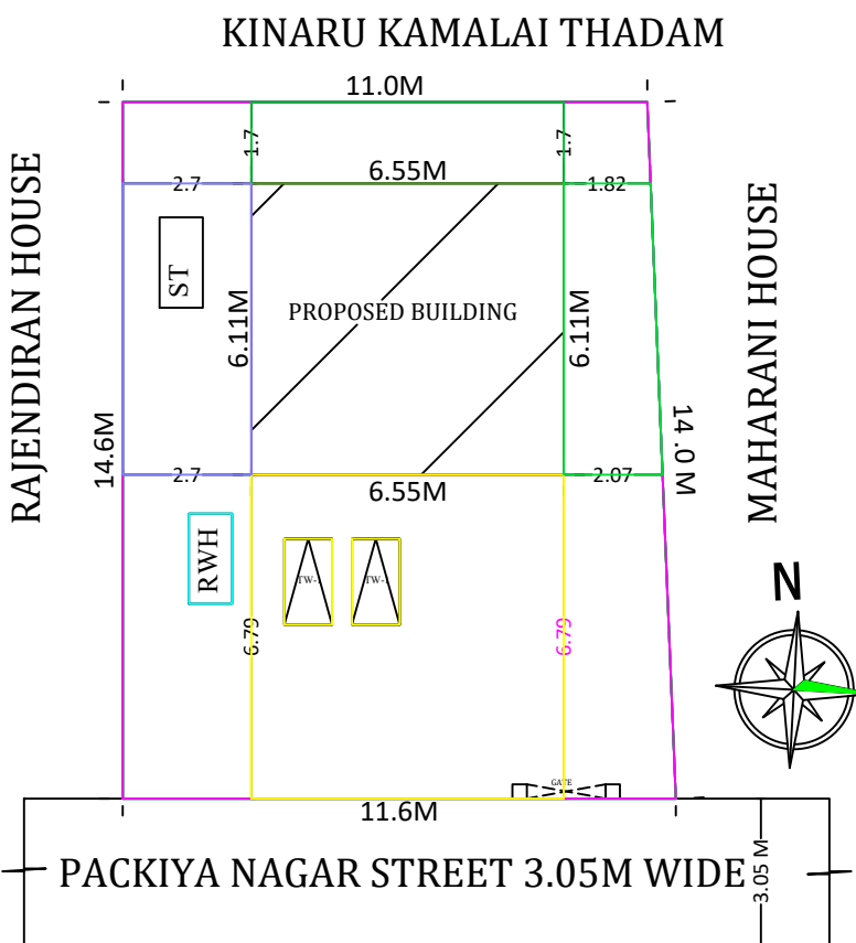
SITE PLAN 1:100 SCALE
