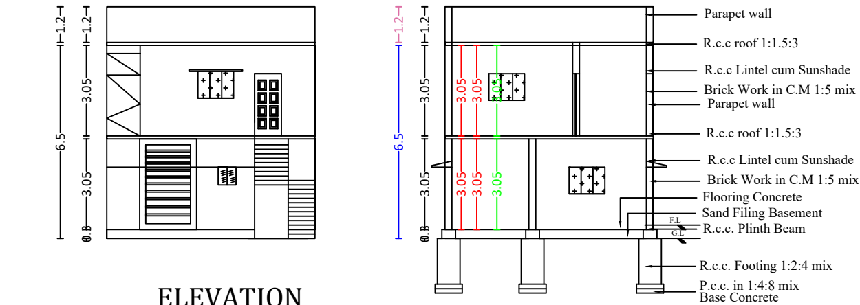
SECTION A-A
