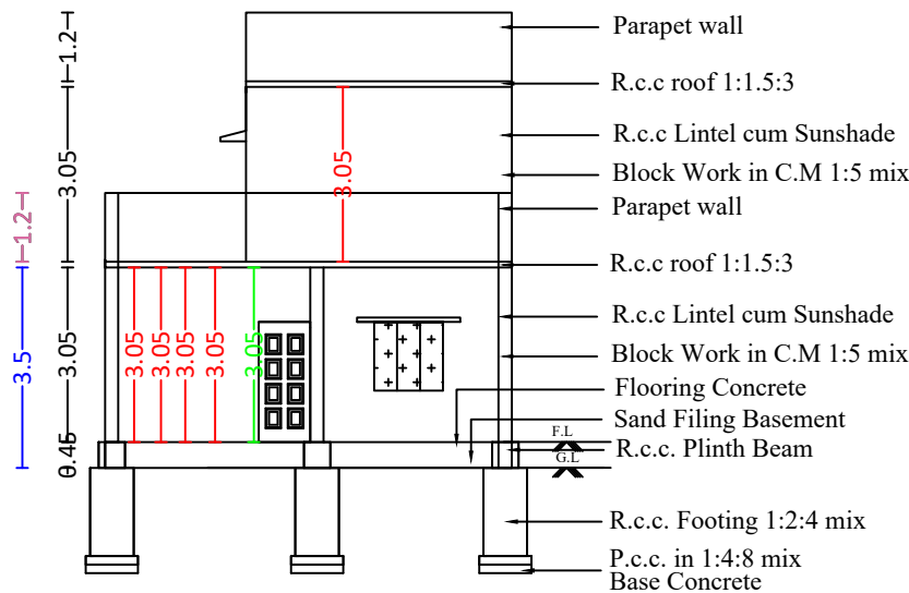
SECTION A-B
