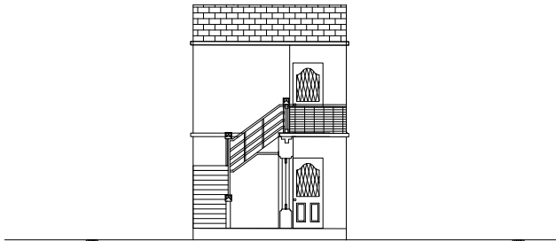
ELEVATION
