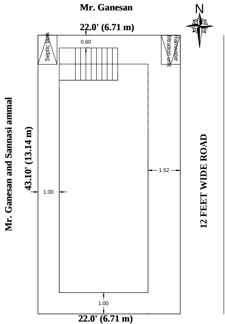
Mr. Ravuthar SITE PLAN
