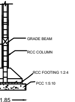
SECTION ON - BB (N.T.S)
