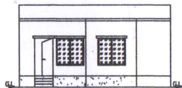
ELEVATION
