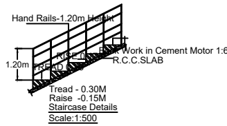
Scale:1:500
