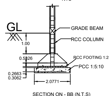
SECTION ON - BB (N.T.S)
