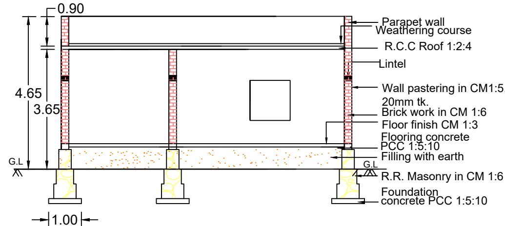
SECTION A-B
