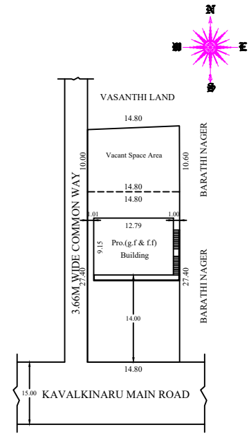
SITE PLAN SCALE 1:400
