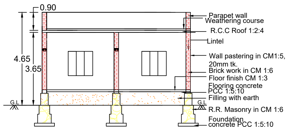
SECTION A-B
