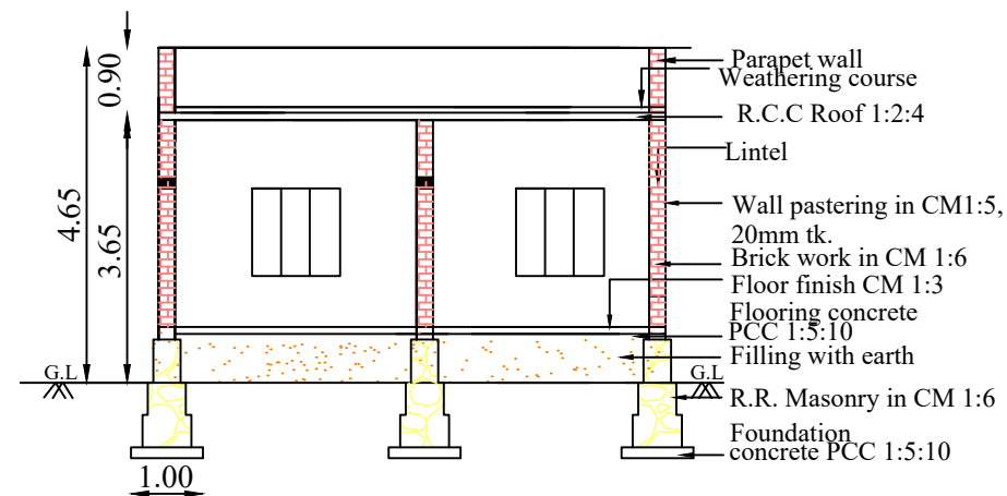
SECTION A-B
