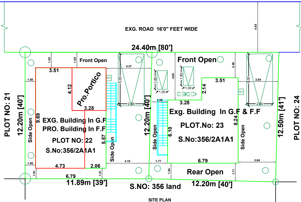
(SCALE 1:100)
