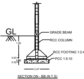
SECTION ON - BB (N.T.S)
