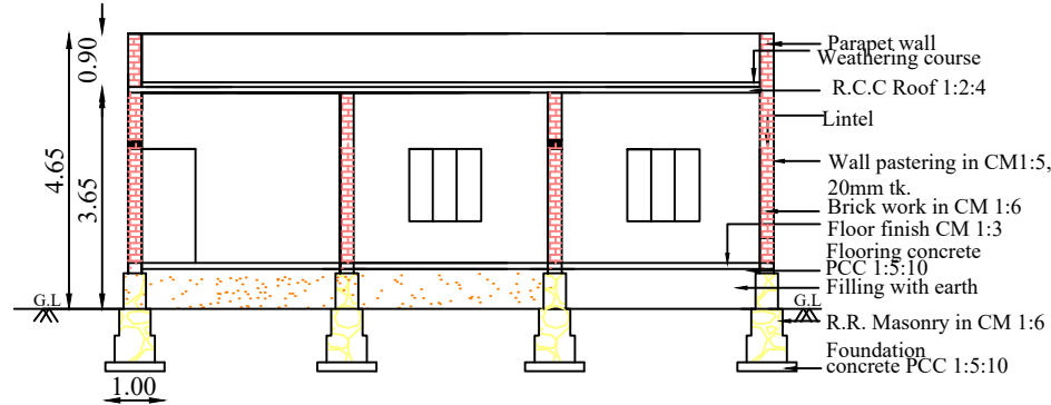
SECTION A-B
