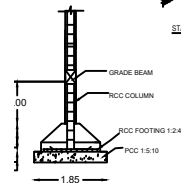
SECTION ON - BB (N.T.S)
