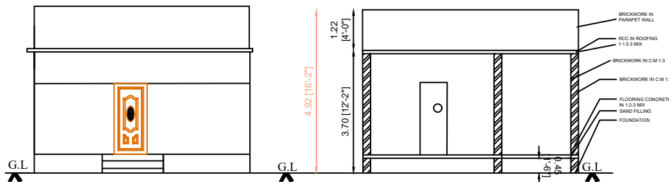
ELEVATION
