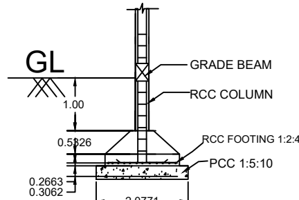
SECTION ON - BB (N.T.S)
