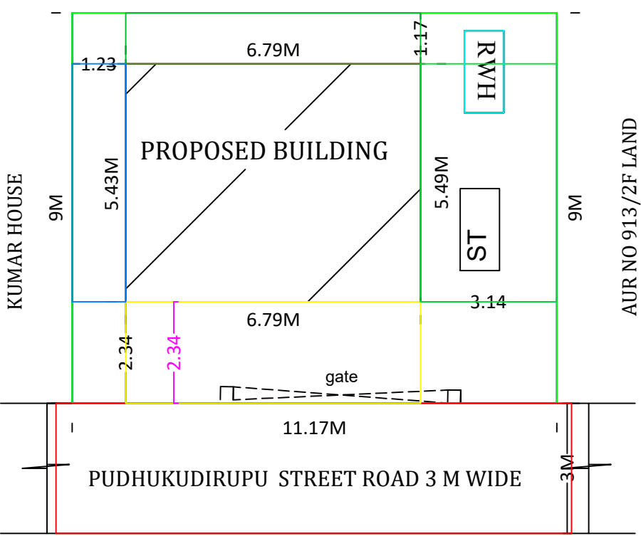
SITE PLAN 1:100 SCALE
