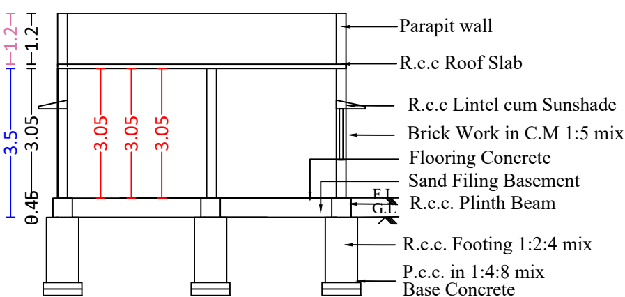
SECTION A-B
