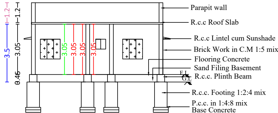
SECTION A-B
