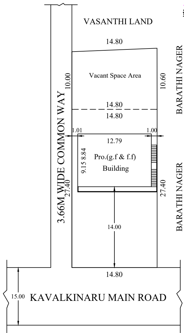
SITE PLAN SCALE 1:400
