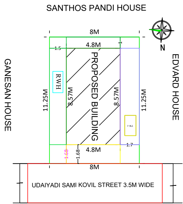
SITE PLAN 1:100 SCALE
