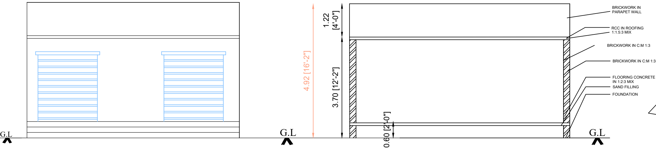
ELEVATION
