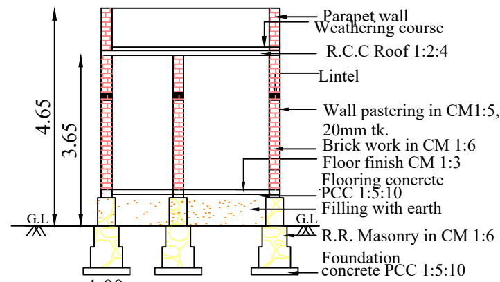
SECTION A-B
