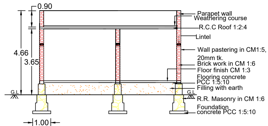
SECTION A-B
